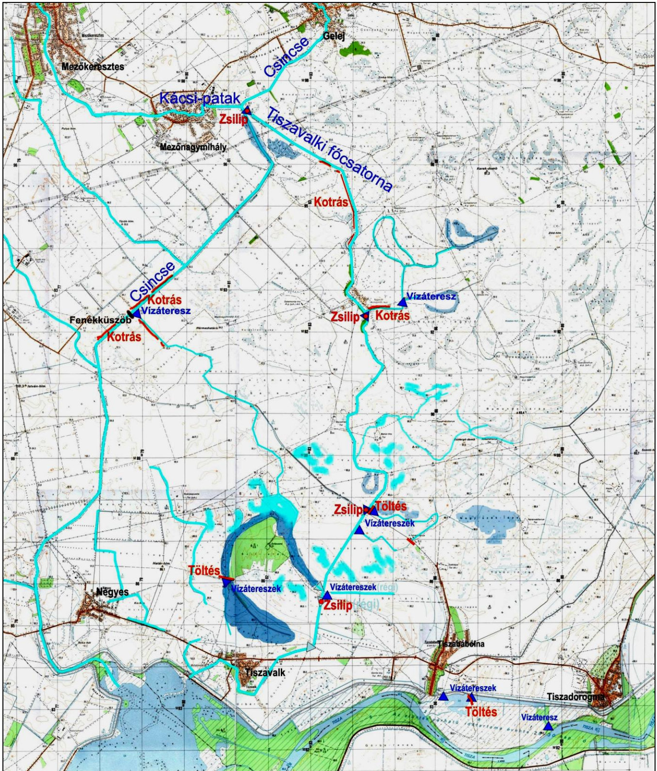
Az I. ütemben elkészült műtárgyak által kormányozhatóvá tett felszíni vízgazdálkodási terület
